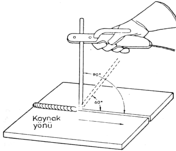
Şekil: 166 - Arkın dikey pozisyonda tutuşturulmasından sonra elektrod 20-30° kadar ilerleme yönünde yatırılabilir. Fazla yatırıldığında püskürme ve gözenek hasil olabilir.
